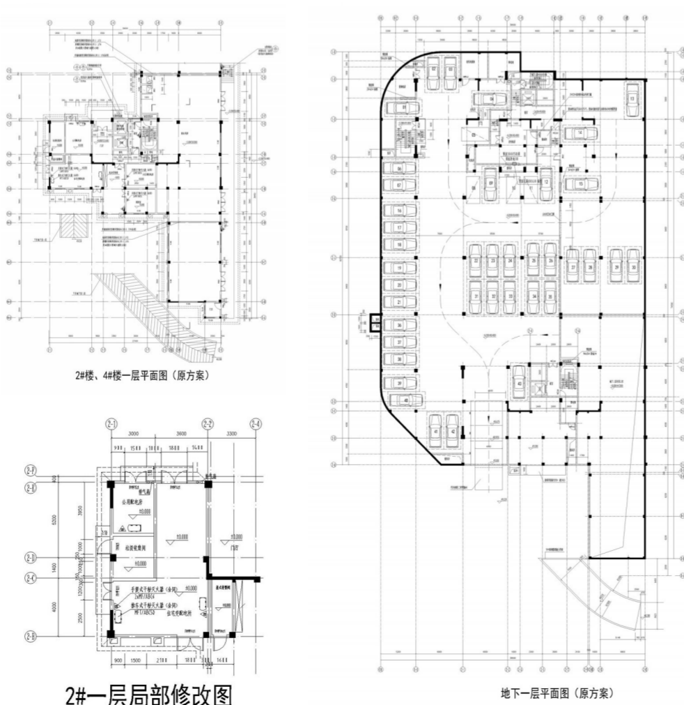
2#一层局部修改图
